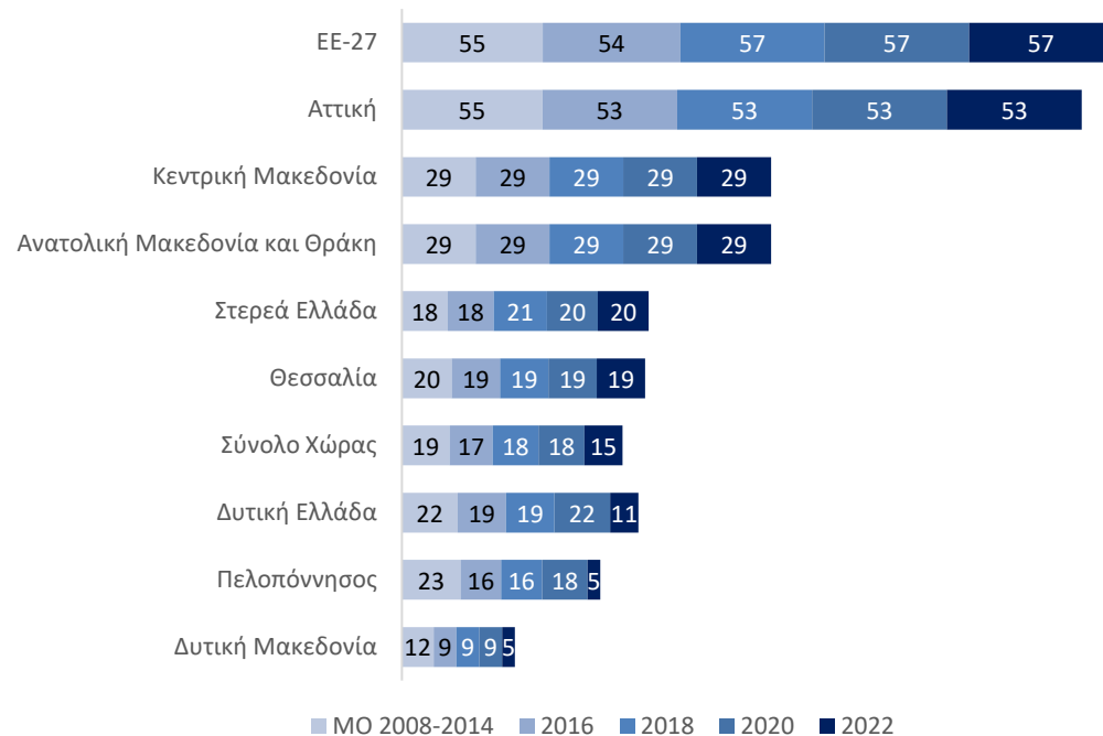
Σιδηροδρομικό δίκτυο (χλμ. σιδηροδρομικών γραμμών ανά χιλιάδες τετραγωνικά χλμ. γης)
